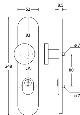
Zylinderüberstand: 6-11 mm
